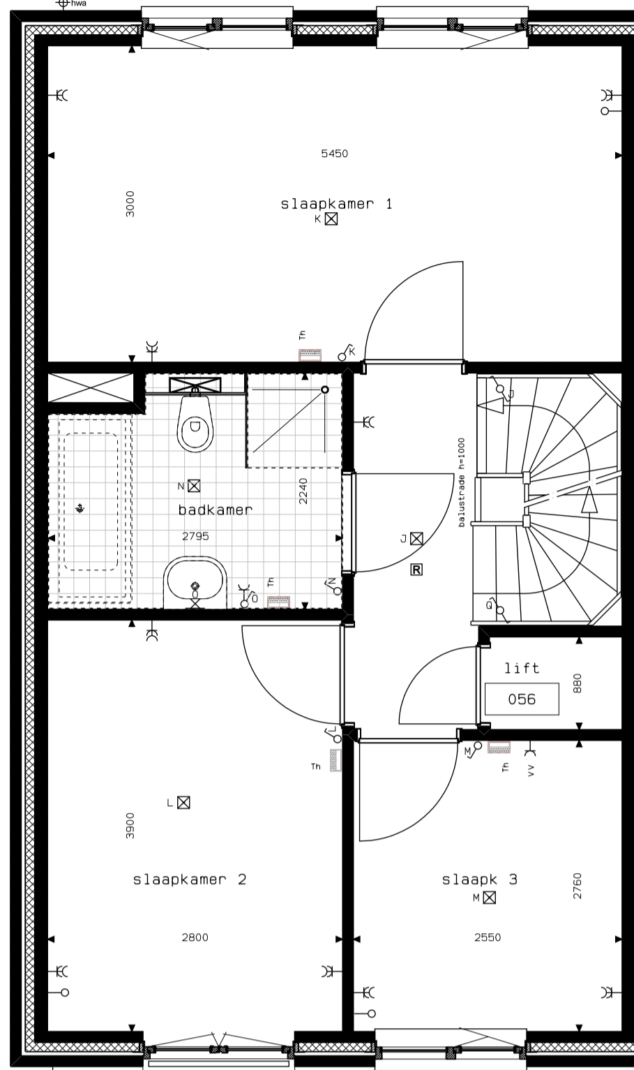
BNR 7,9 BNR 8,10 gespiegeld 1E VERDIEPING
