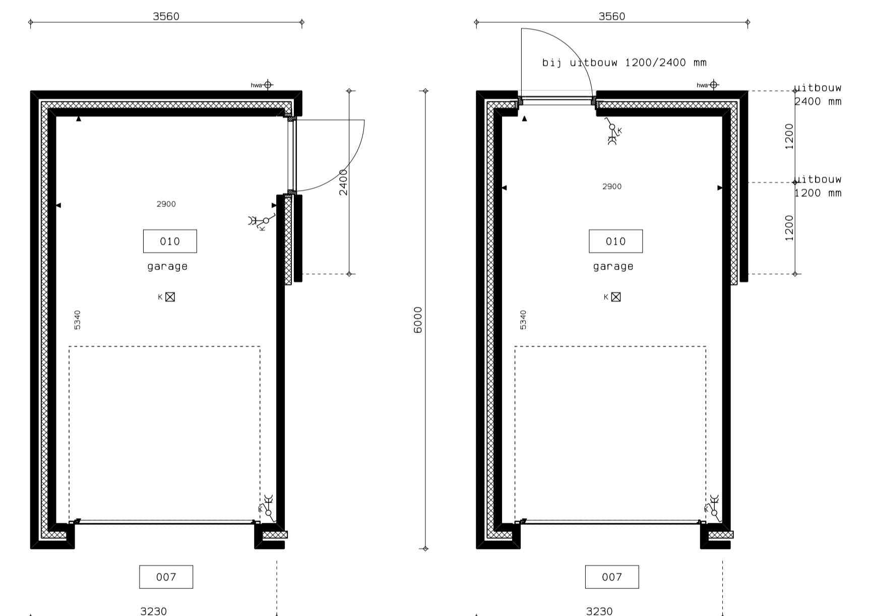
BNR 7,9 BNR 8,10 gespiegeld 1E VERDIEPING
