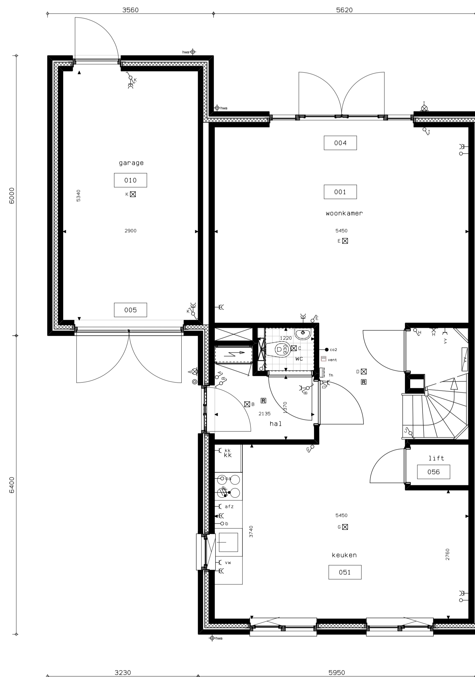
BNR 7,9 BNR 8,10 gespiegeld BEGANE GROND
