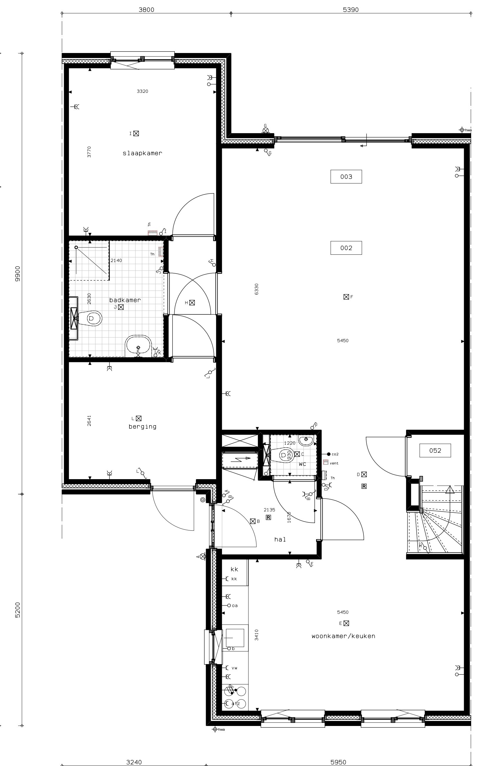
BNR 1, 3, 5 BNR 2, 4, 6 gespiegeld BEGANE GROND
