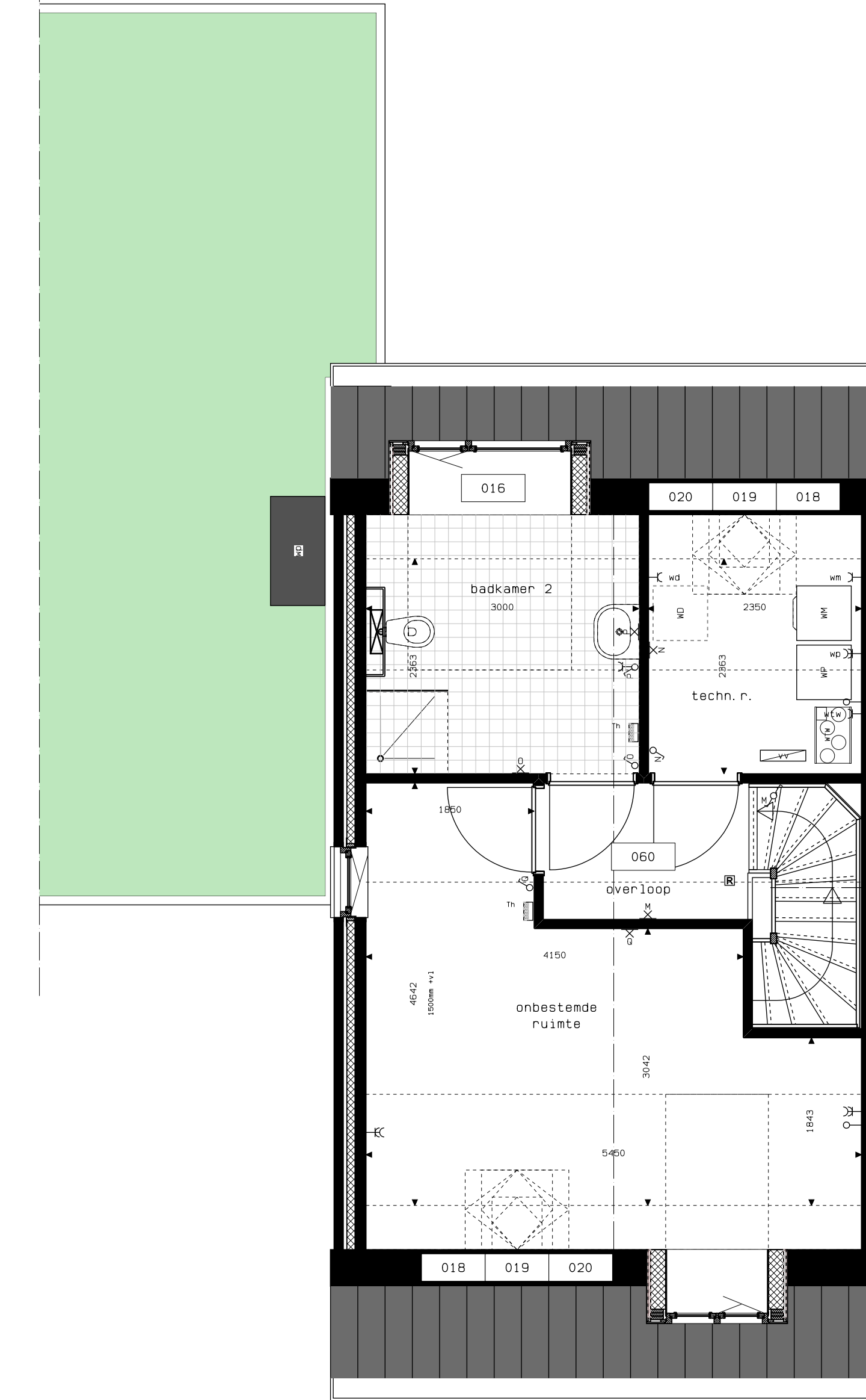
BNR 1, 3, 5 BNR 2, 4, 6 gespiegeld 1E VERDIEPING
