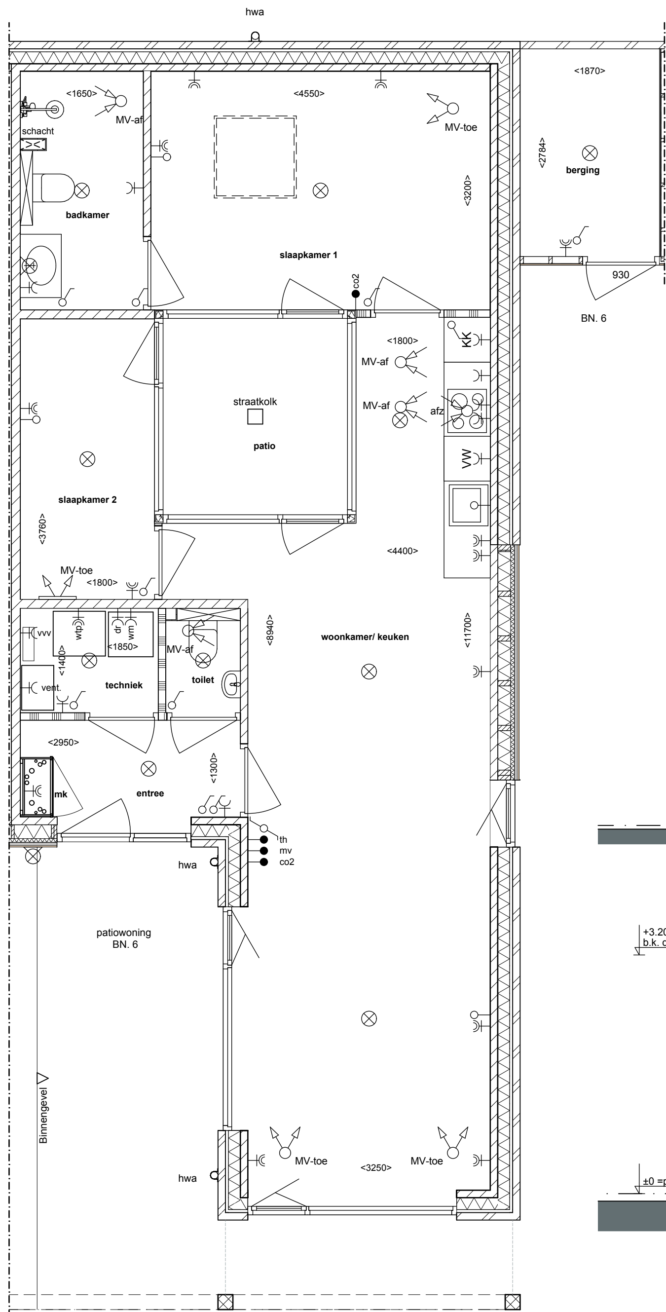
Begane grond - 1:50
