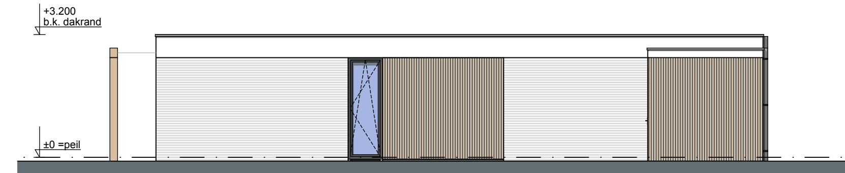
Rechter zijgevel - 1:100 BN. 6
