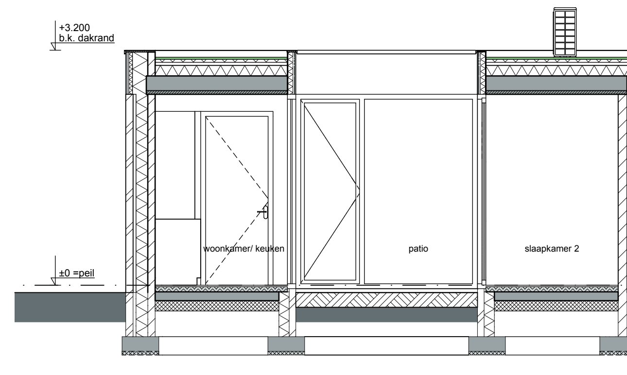
Doorsnede patio - 1:50 BN. 1
