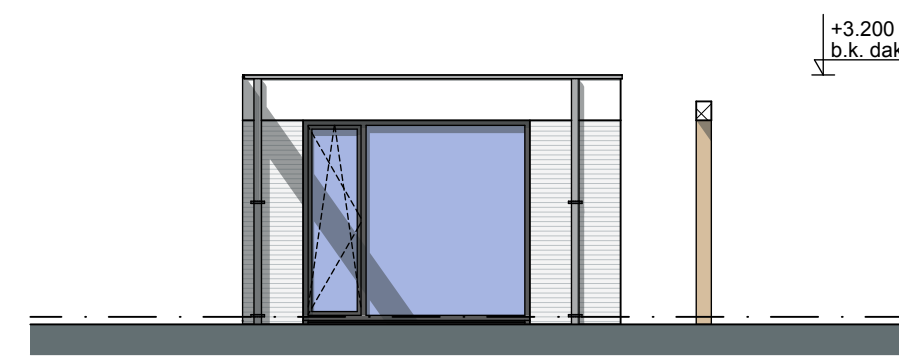
Binnengevel - 1:100 BN. 6
