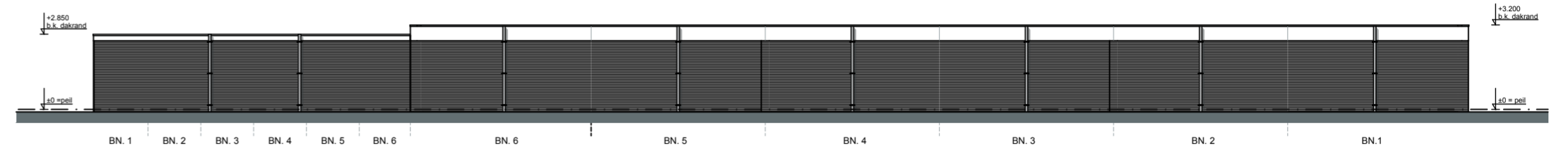
Achtergevel - 1:200
