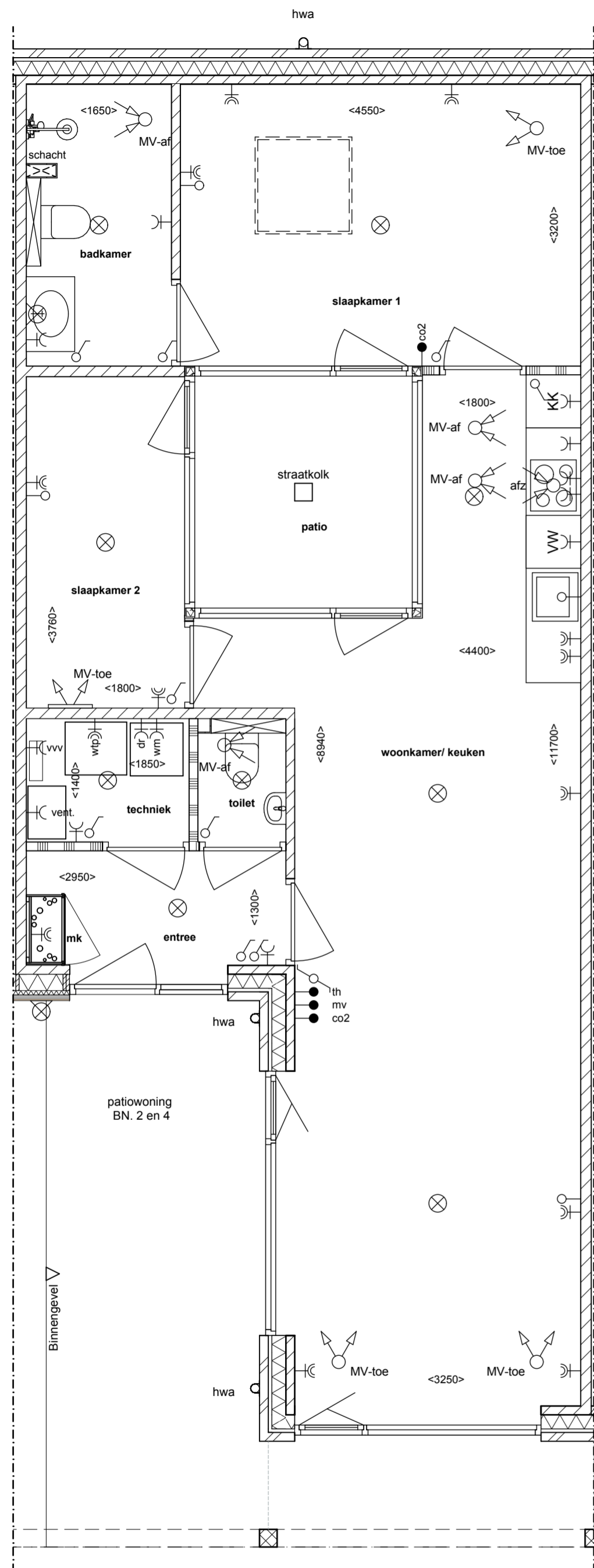
Begane grond - 1:50
