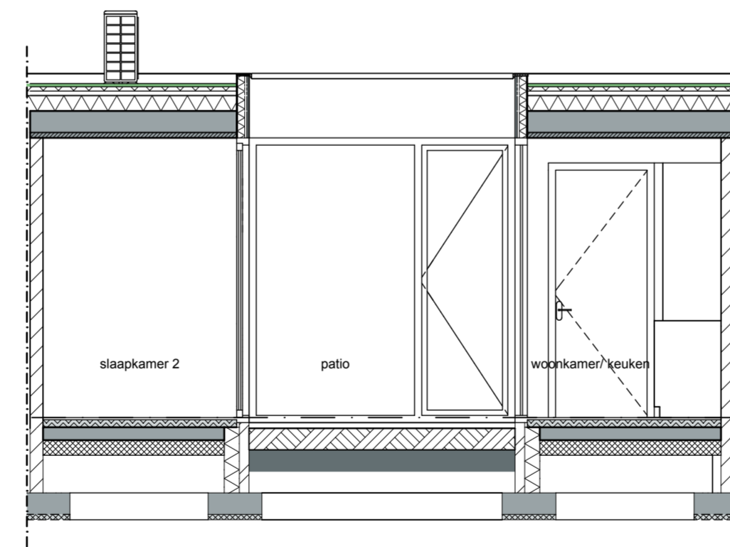
Doorsnede patio - 1:50
