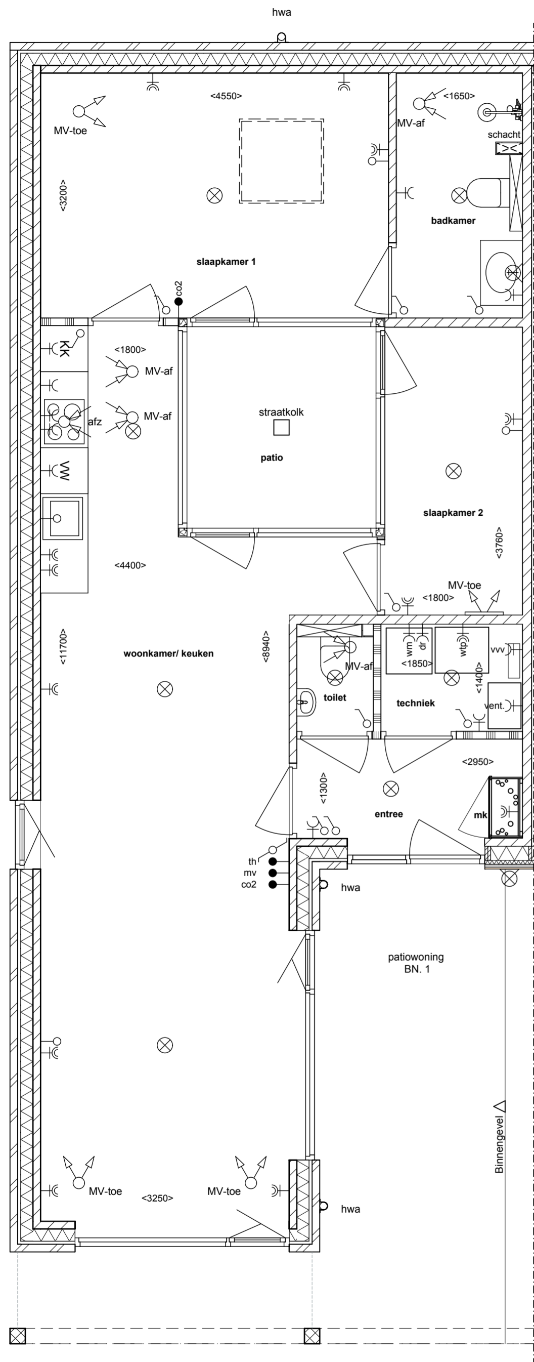
Begane grond - 1:50
