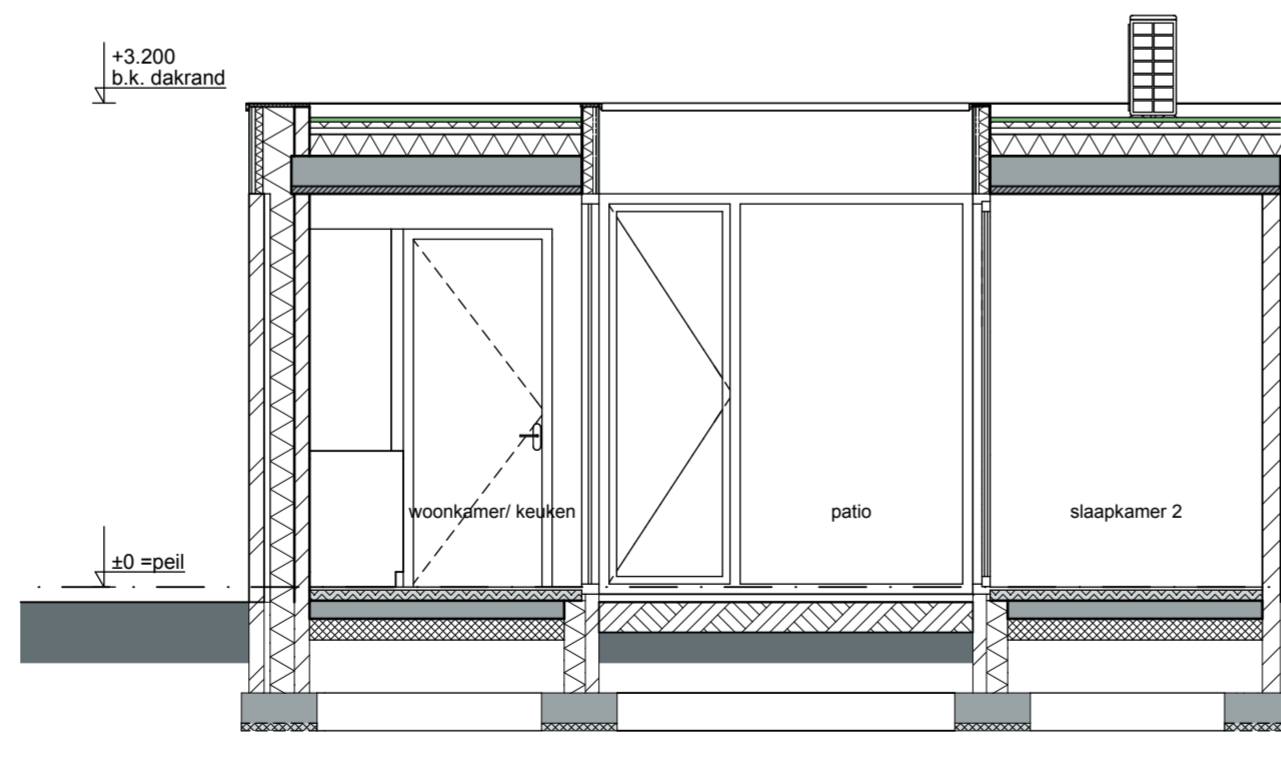
Binnengevel - 1:100
