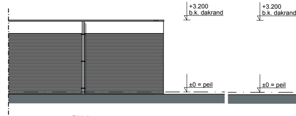
Achtergevel - 1:100
