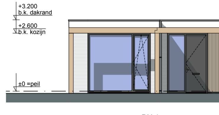
Voorgevel - 1:100
