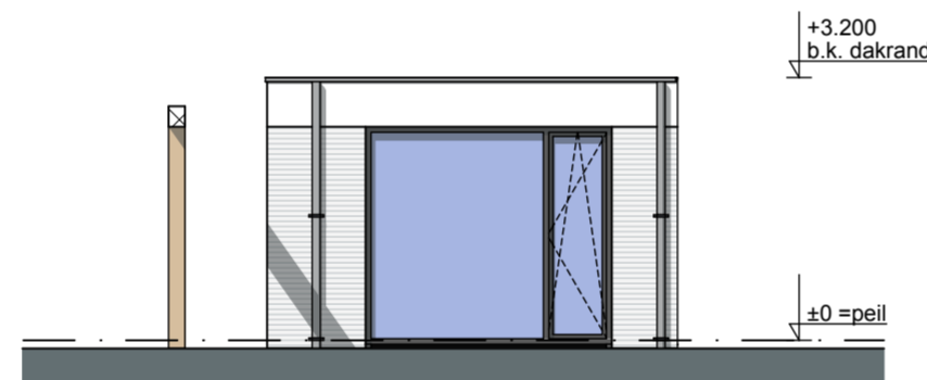
Binnengevel - 1:100
