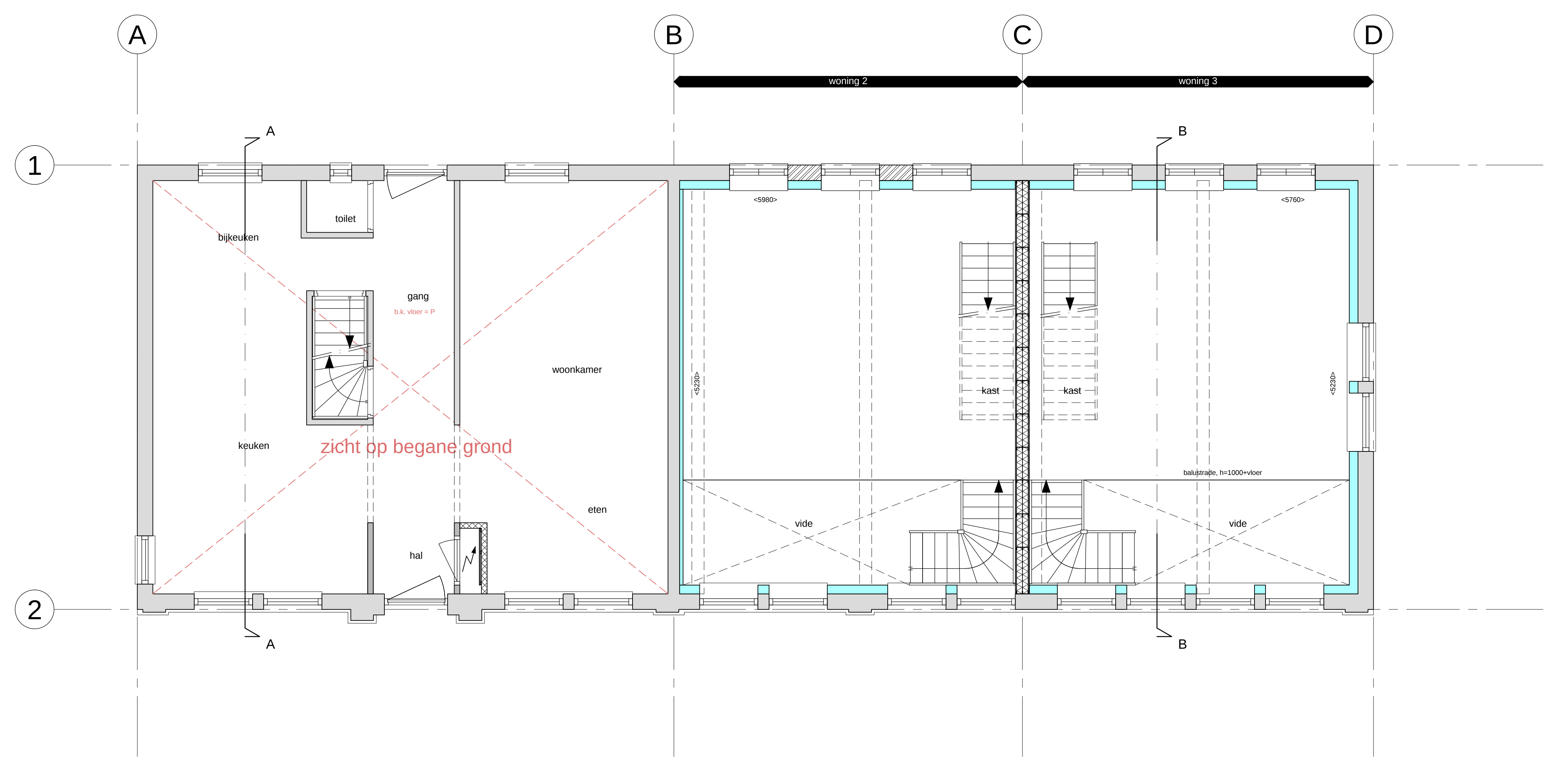
tussenverdieping (1:50)
