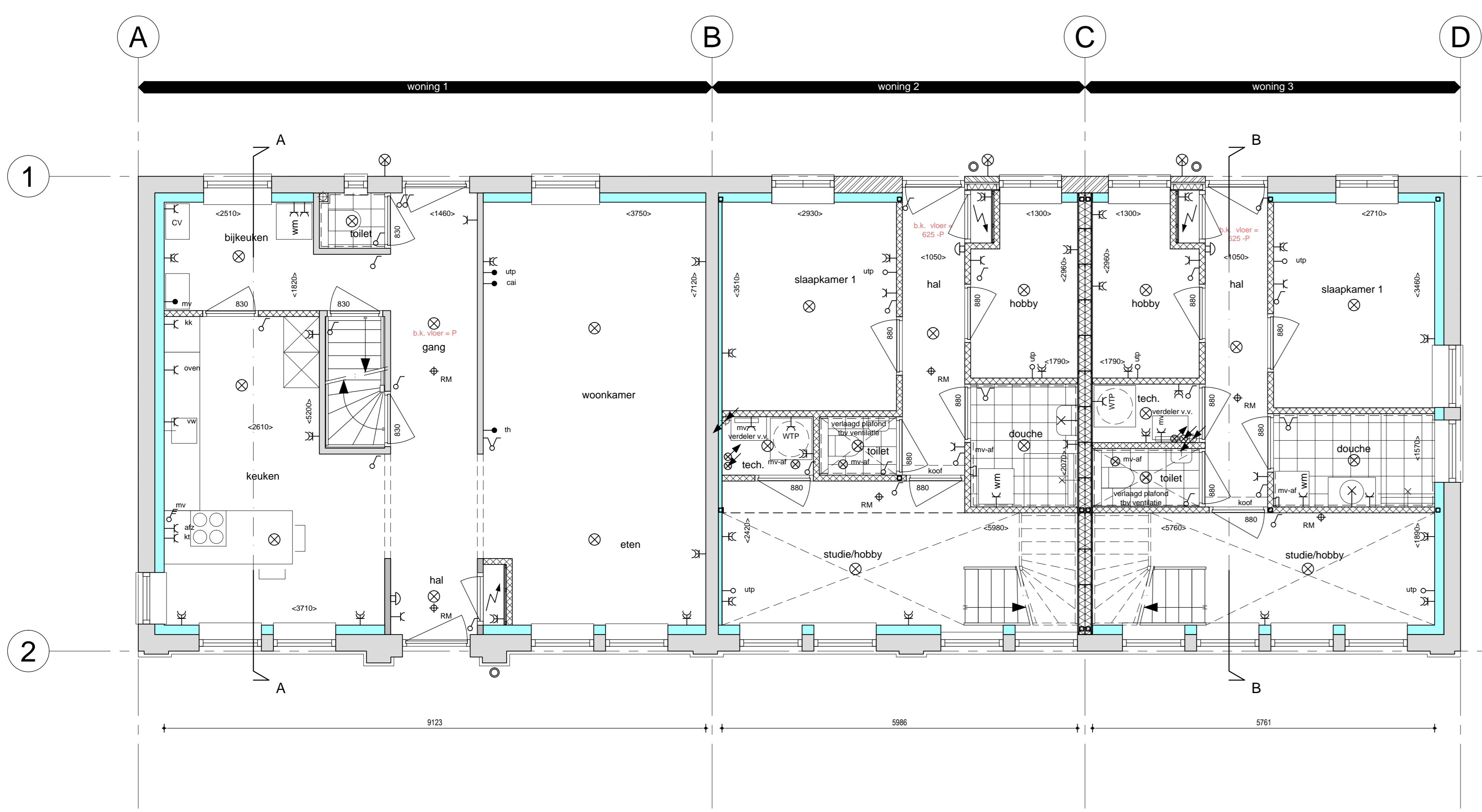
begane grond (1:50) RM ⌘ = rookmeter MV ⌘ = mechanische afvoer ventilatie ⌘ = dakramen met ventilatie ⌘ = waswastap
