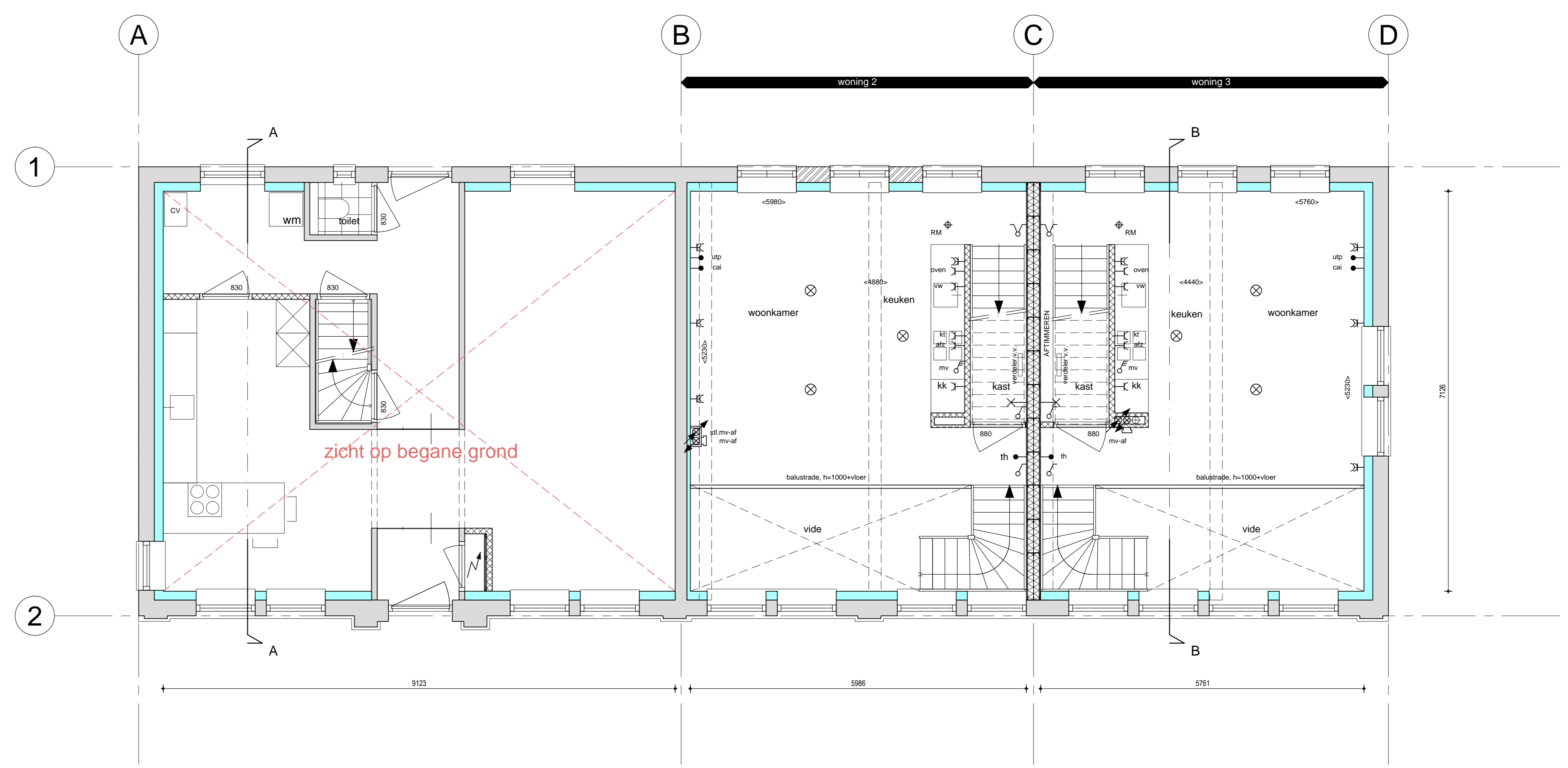
tussenverdieping (1:50) RM ⌘ = rookmeter MV ⌘ = mechanische afvoer ventilatie ⌘ = dakramen met ventilatie ⌘ = waswastap
